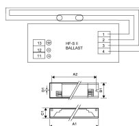
Caractéristiques Philips HF-S 158 TL-D II 50/60Hz
